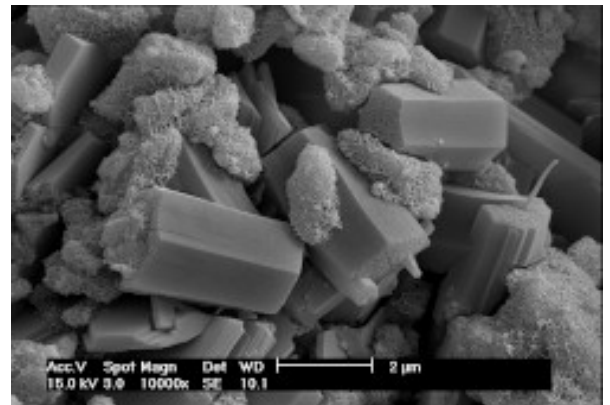
Hydratatie van Ultracolor Plus speciaal bindmiddel op cementbasis. Let op de afwezigheid van lamellaire Portlandiet kristallen (calcium hydroxide), die de oorzaak zijn van witte uitslag
